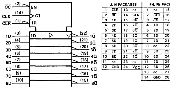
logic symbol, 'ALS577, 'AS577
